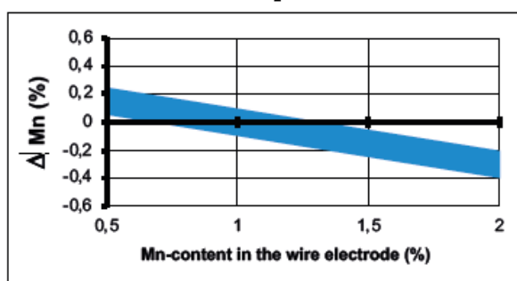
Absorción o deposición de Mn
