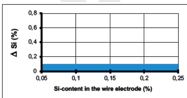
Absorción de silicio
